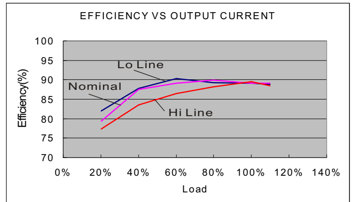
SU-2405S12
