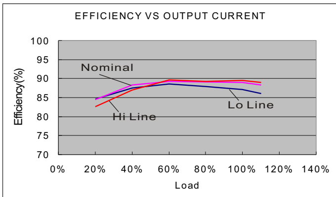
SU-1205S12
