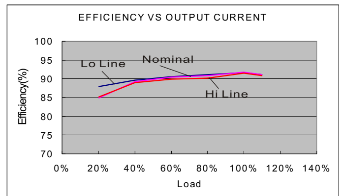
SU-2415D12
