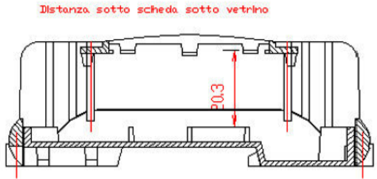
Sez. H-H
