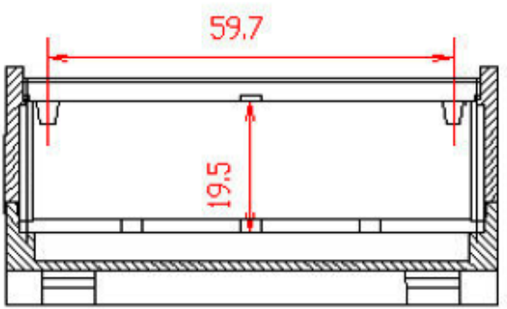
Sez. G-G
