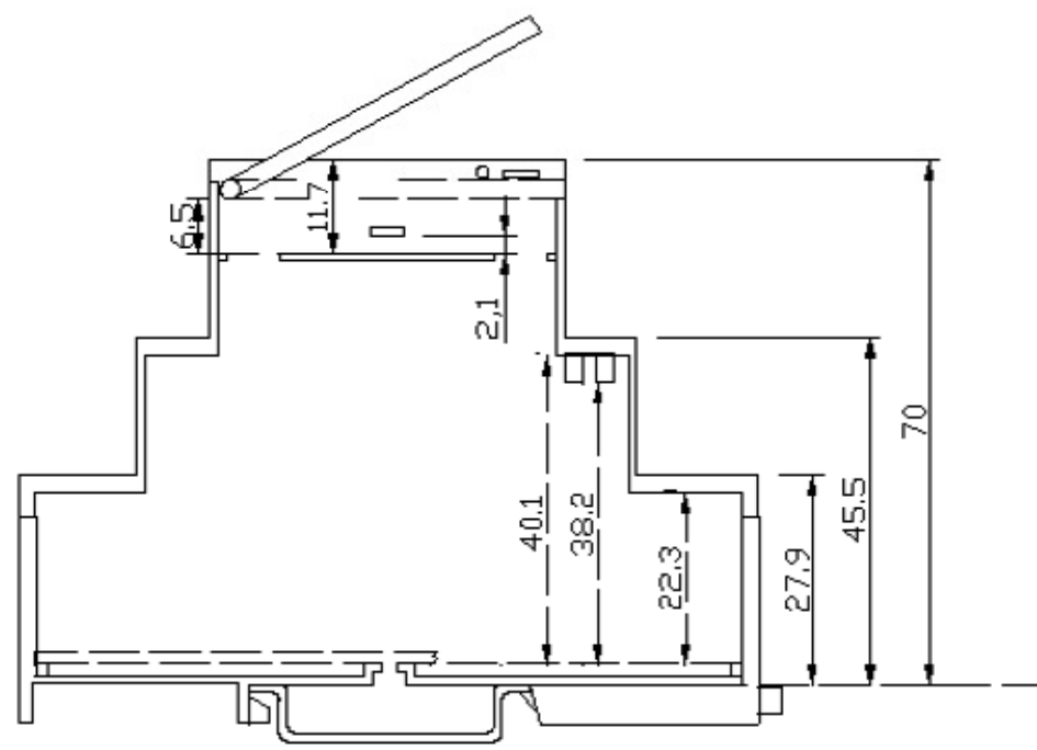
BARRA DIN
