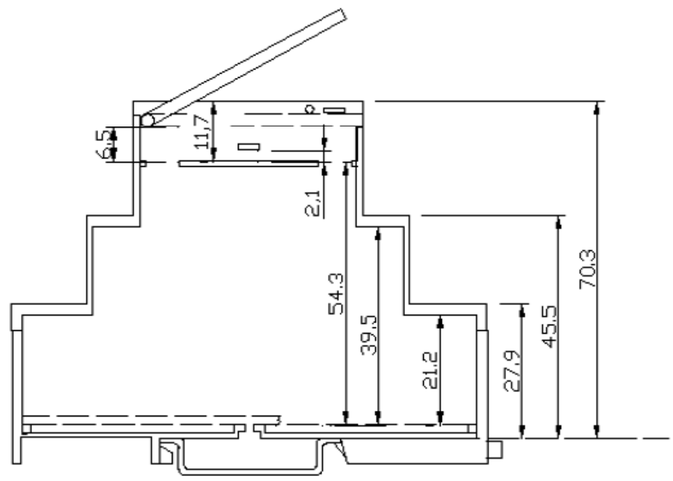
BARRA DIN
