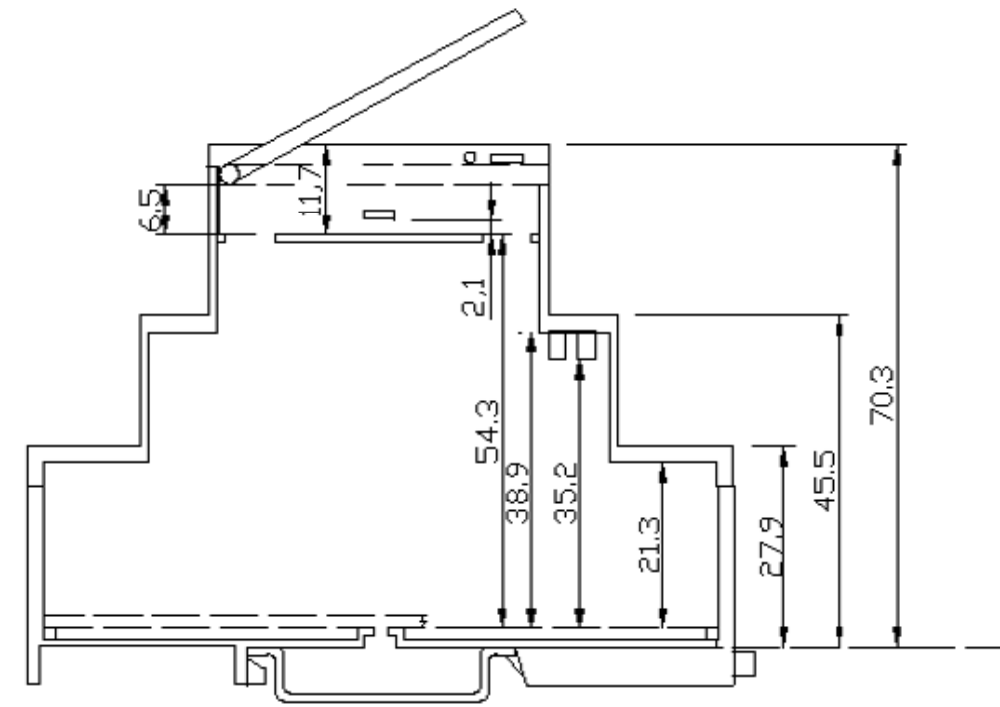
BARRA DIN
